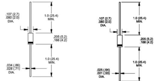
DO-204AL (DO-41)
