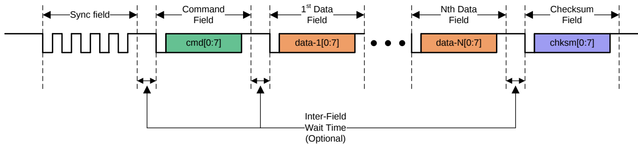
图 22. UART Interface Transmission Frame
