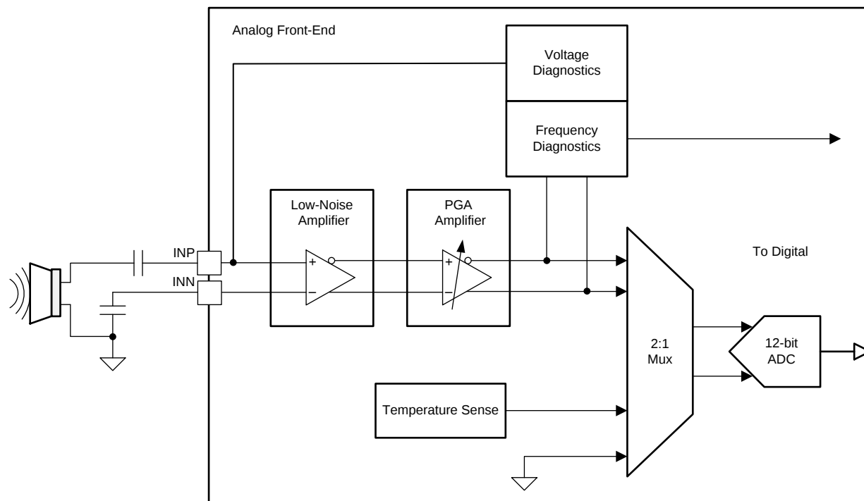
图 5. Analog Front-End
