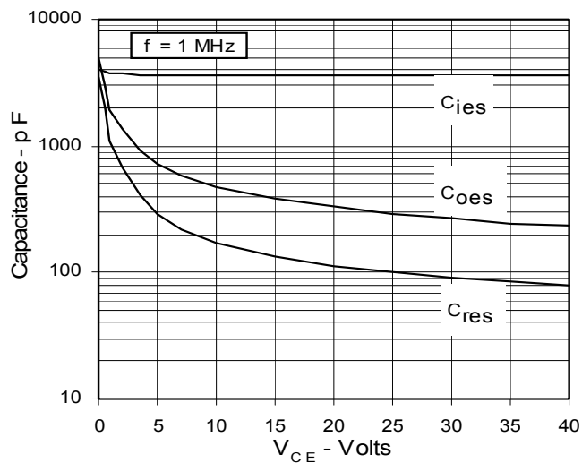
Fig. 15. Capacitance
