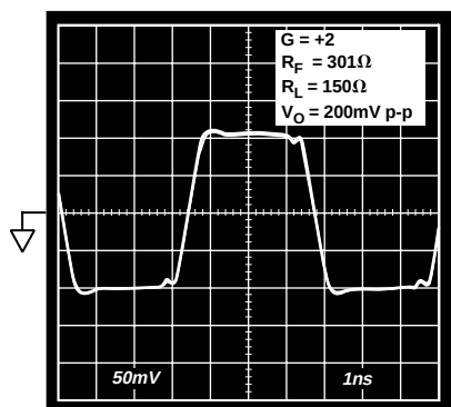
TPC 27. 2 V瞬态响应; G = +2
