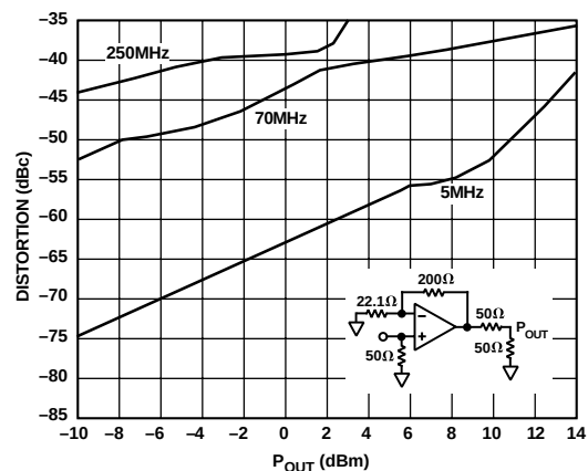
TPC 10. 二次谐波失真与 P_{OUT} 的关系; ( G = +10 )
