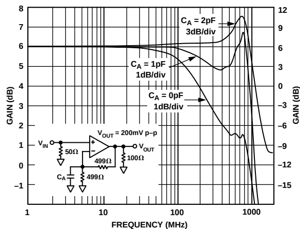
TPC 35. 小信号频率响应与寄生电容的关系
