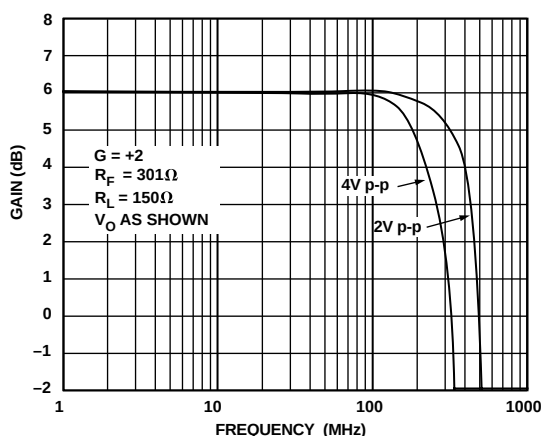
TPC 2. 大信号频率响应; G = +2
