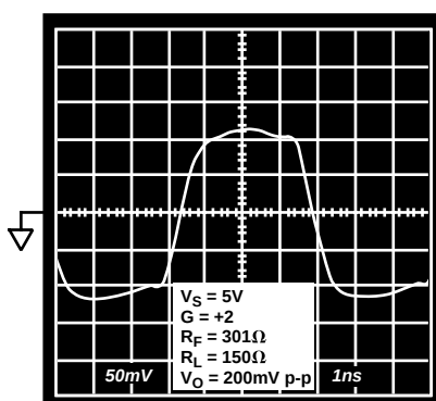
TPC 33. 小信号瞬态响应; V_S = 5\text{ V} ; G = +2
