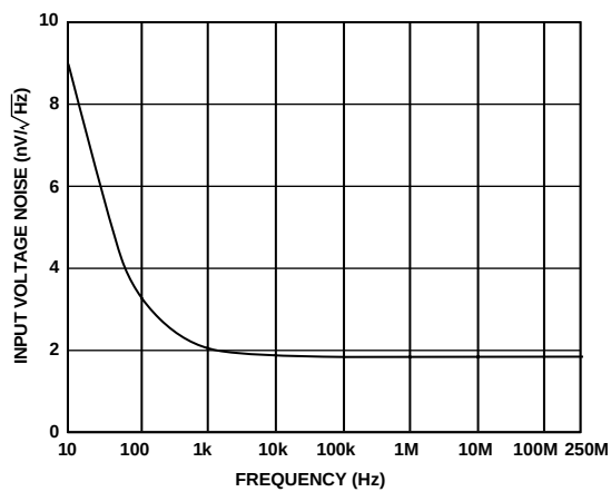
TPC 20. 电压噪声与频率的关系
