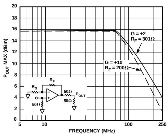
TPC 23. 最大输出功率与频率的关系
