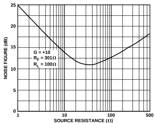
TPC 21. 噪声系数
