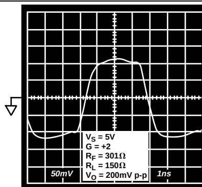
TPC 34. 2 V瞬态响应; V_S = 5\text{ V} ; G = +2
