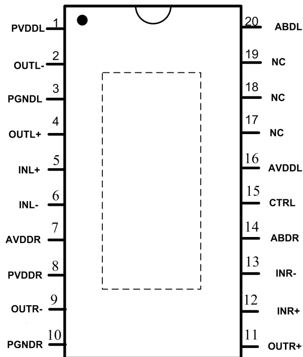
HT8697 顶视图
