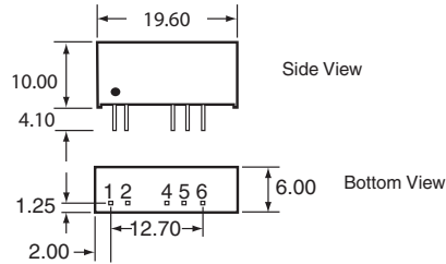
CTDD1906SF-D1K-1 Package
