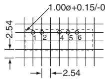
CTDD1906SF-D1K-1 Footprint
