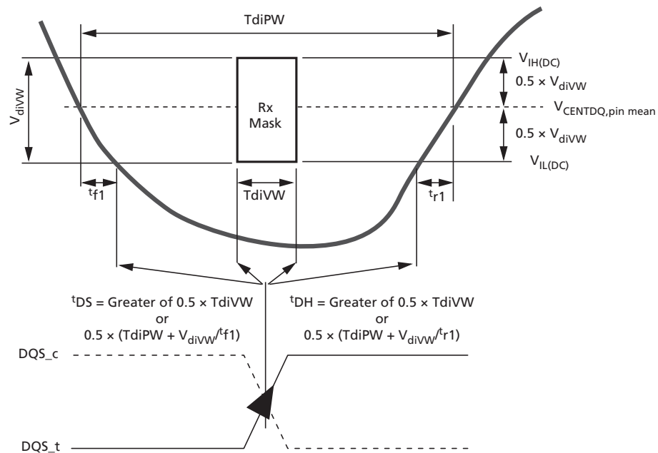
Figure 207: Rx Mask Relative to t DS/ t DH
