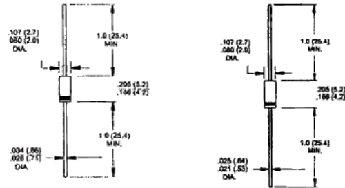
DO-204AL (DO-41)
