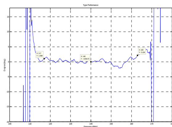
Phase Linearity( f_0 \pm 23\text{MHz} )
