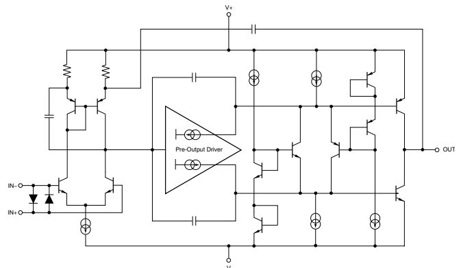
功能方框图
