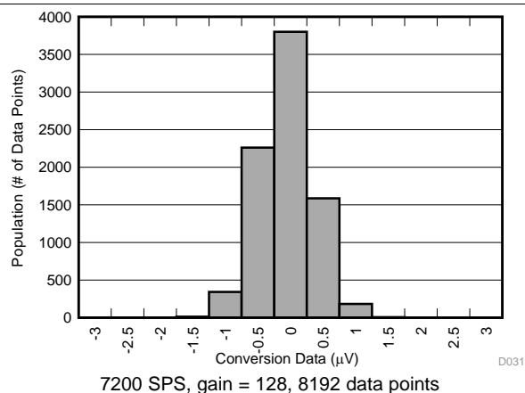
图 25. Conversion Data Histogram
