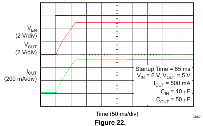
STARTUP
