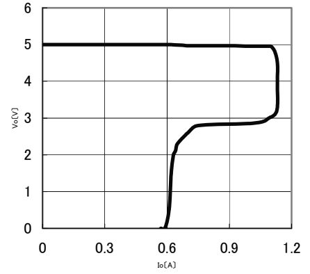
Fig.15 OCP
