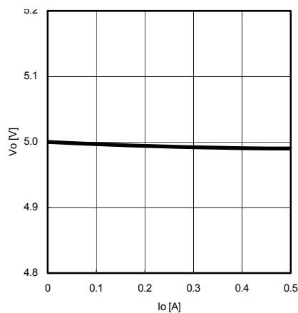
Fig.11 I_o - V_o
