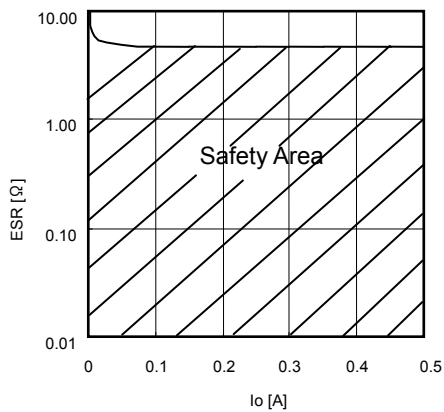
Fig.17 ESR condenser
