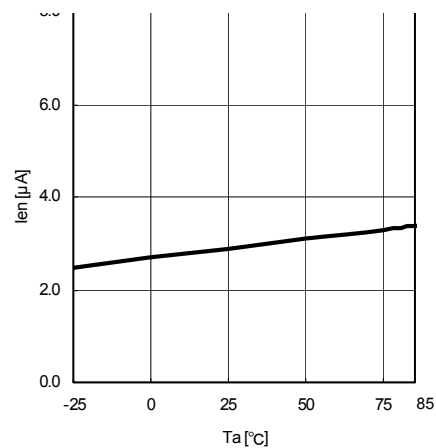
Fig.10 T_a - I_{EN}
