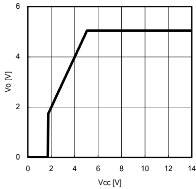
Fig.13 V_{cc}-V_o ( I_o=0\text{mA} )
