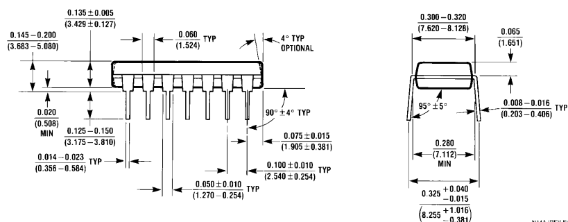
N14A (REV F)
