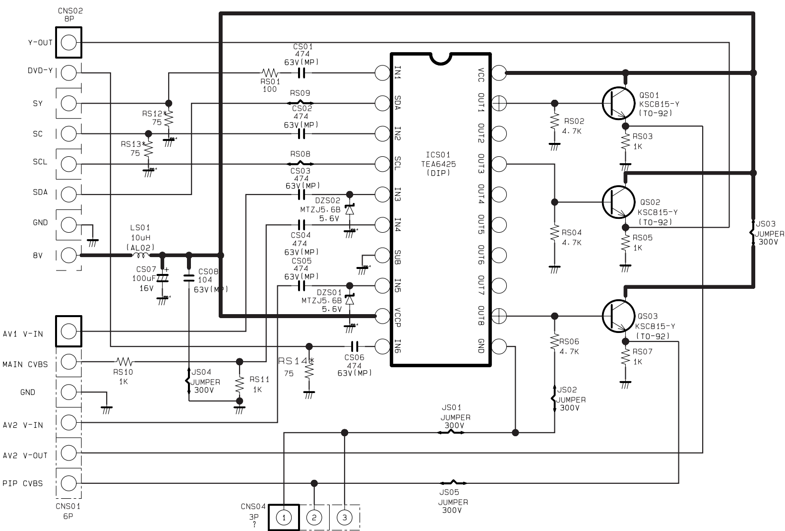
KS2A/KS3A VIDEO S/W MODULE (TEA6425)
