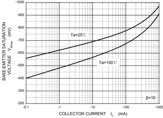
V_{BE} - I_c
