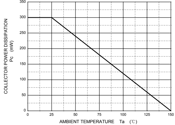
P_c - T_a
