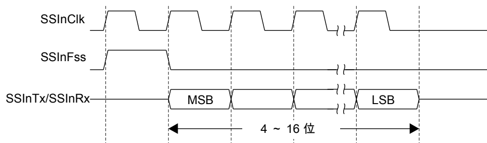
图 14-2. TI 同步串行帧格式 (单次传输)
