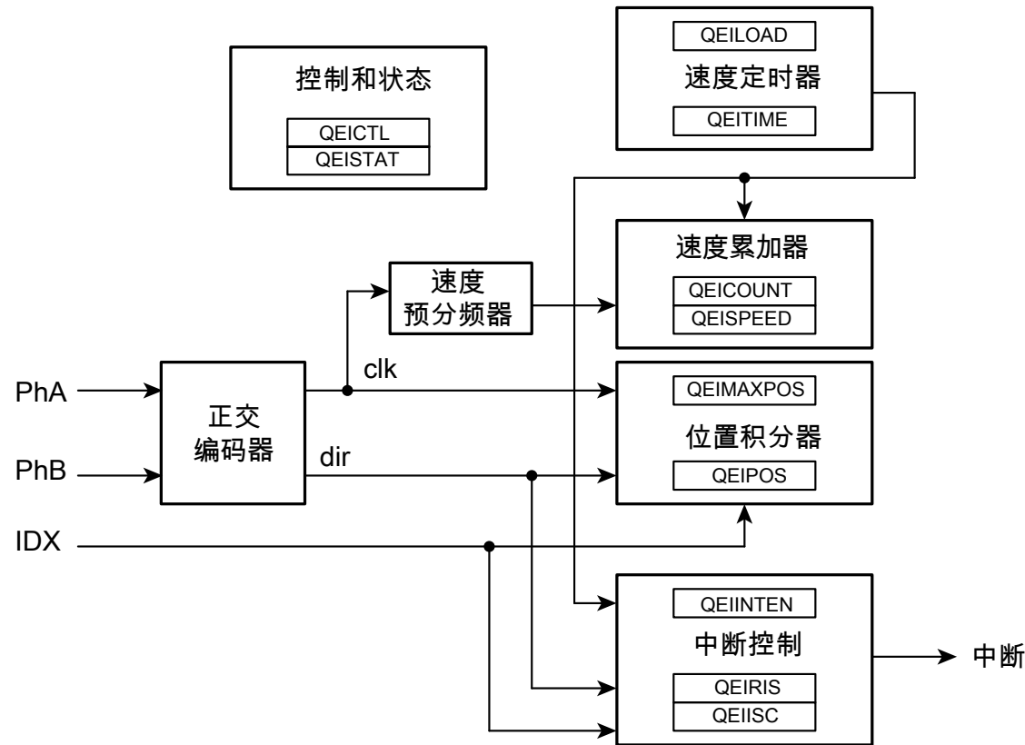
图 19-1. QEI结构图
