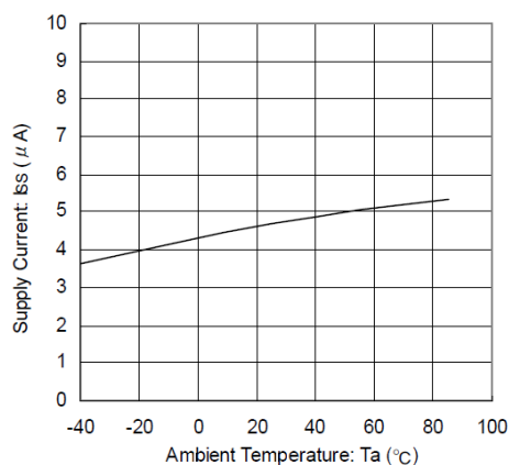
IXD1216B/D 332xx
