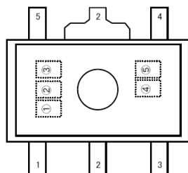
SOT-89-5
