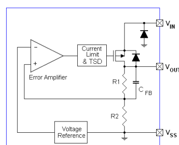
IXD1216D
