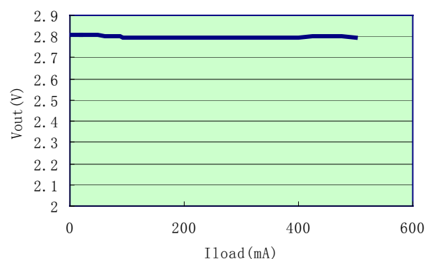
LR8558-2.8V Output
