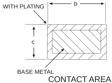
14 PIN NSOIC
