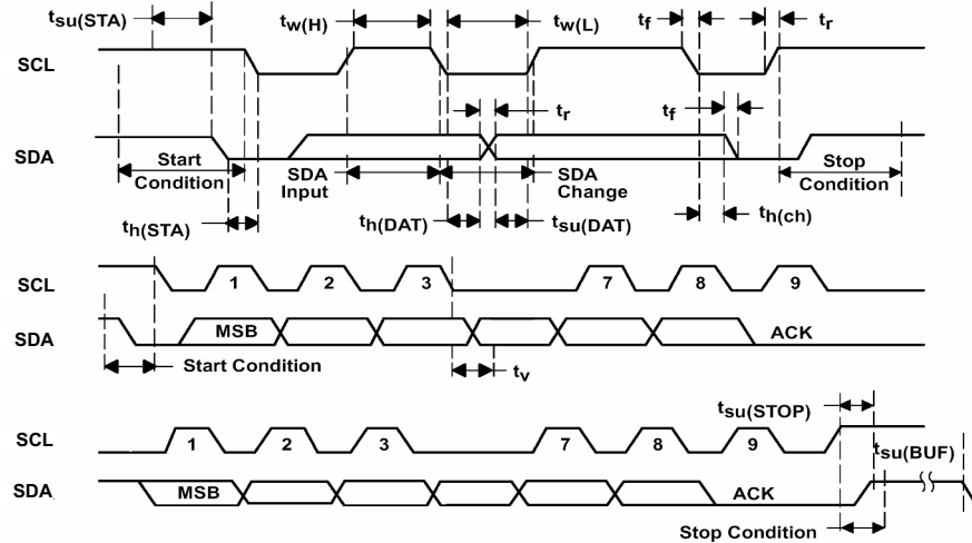
图 7-1. I²C Timing
