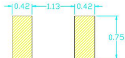
推荐焊盘尺寸
