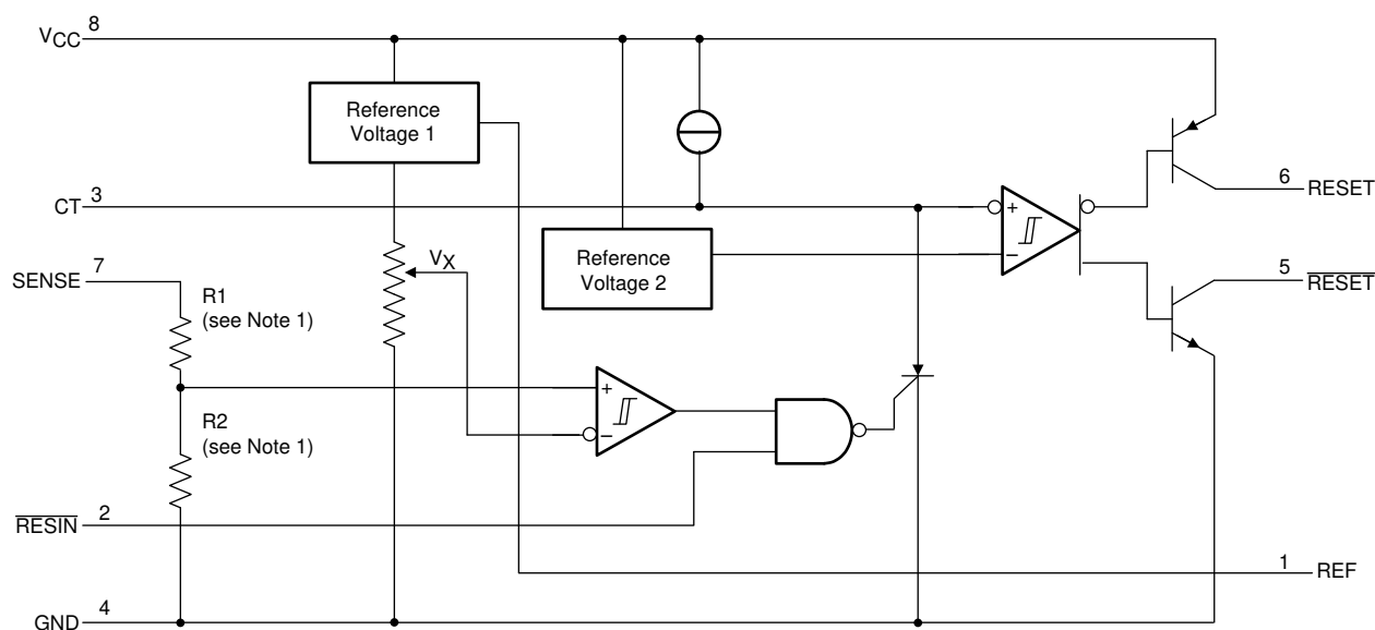
功能方框图
