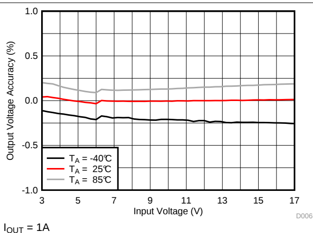
图 21. Line Regulation
