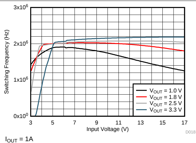
图 23. Switching Frequency
