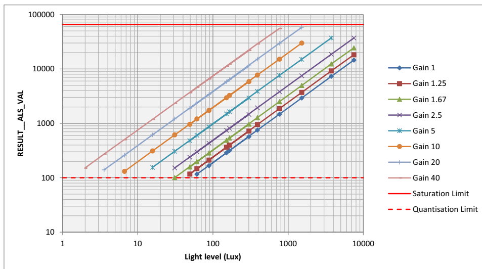
Figure 7. ALS linearity
