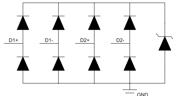
TPD4E05U06-Q1 框图
