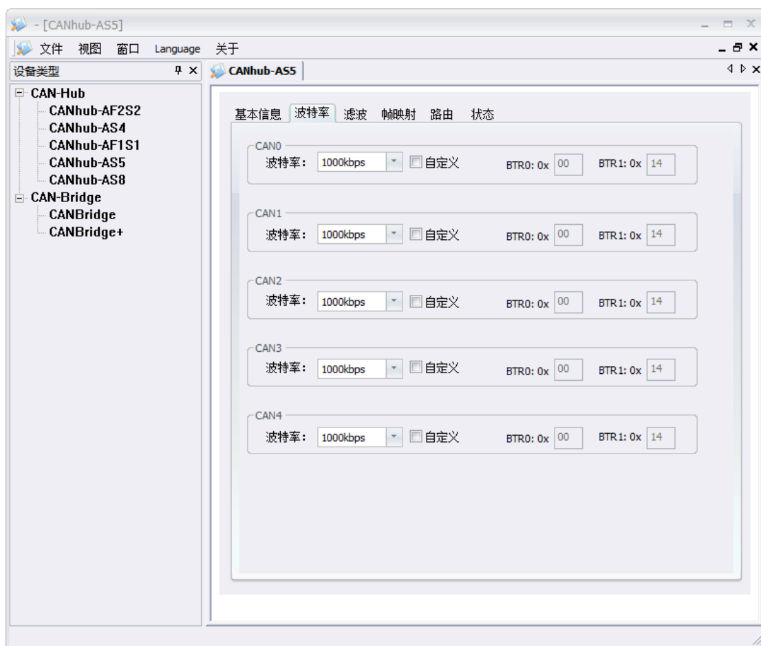
图 4.5 波特率窗口
