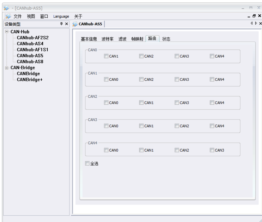
图 4.13 路由窗口
