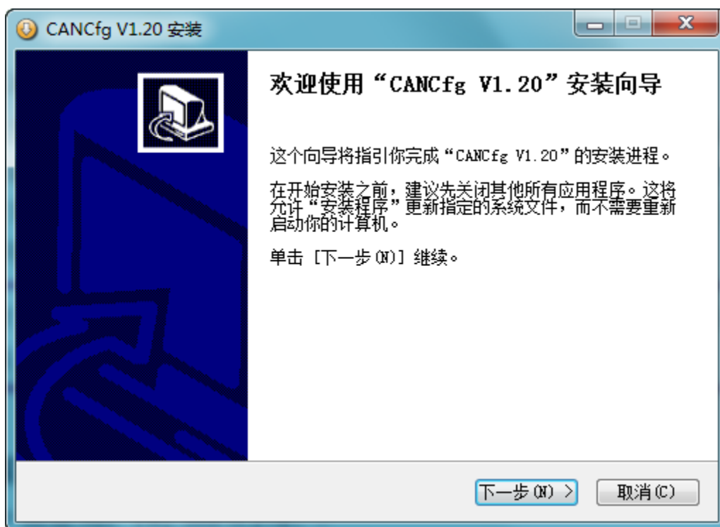
图 3.1 欢迎界面
