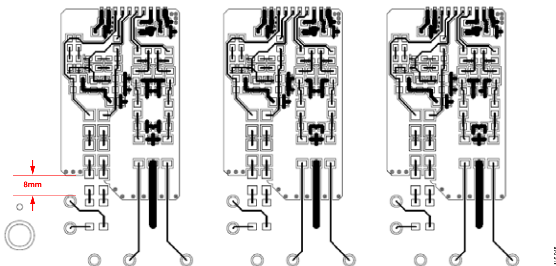
图57. 4层电路板：顶层
