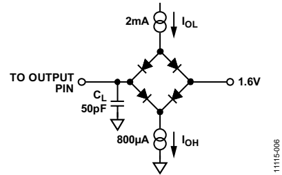
图 6. 时序规格的负载电路
