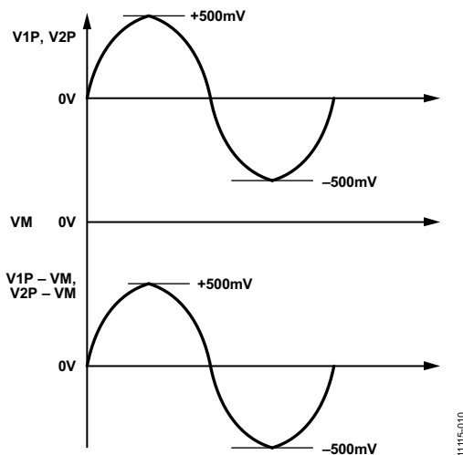
图22. V1P和VM引脚之间以及V2P和VM引脚之间的伪差分输入电压范围
