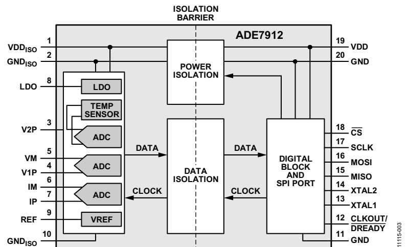
图2. ADE7912功能框图
