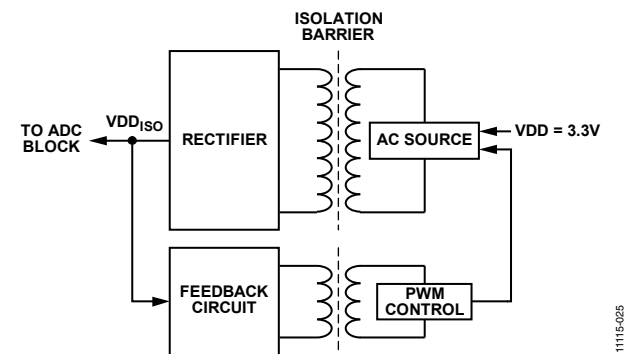
图47. 隔离式DC/DC转换器框图
