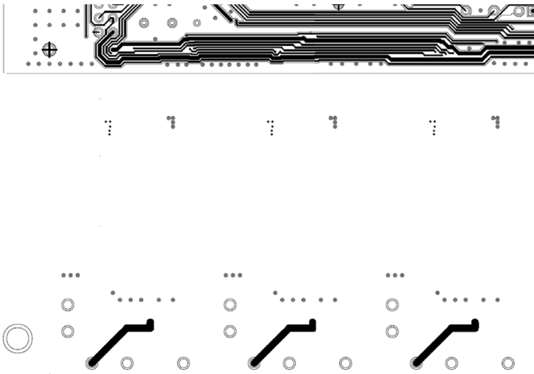
图58. 4层电路板：底层
