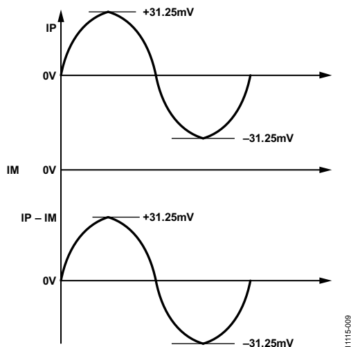
图21. IP和IM引脚之间的伪差分输入电压范围
