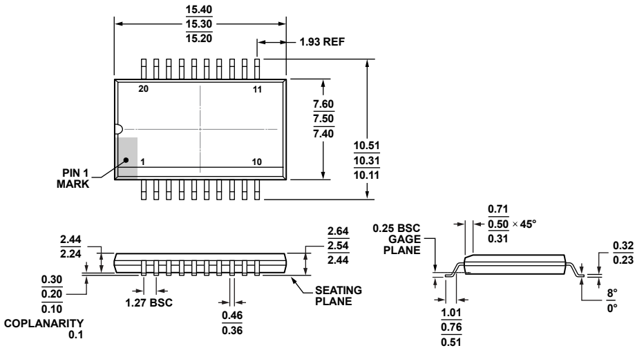
图62. 20引脚标准小型封装，具有增强的爬电性能[SOIC_IC] 宽体 (RI-20-1) 图示尺寸单位：mm
