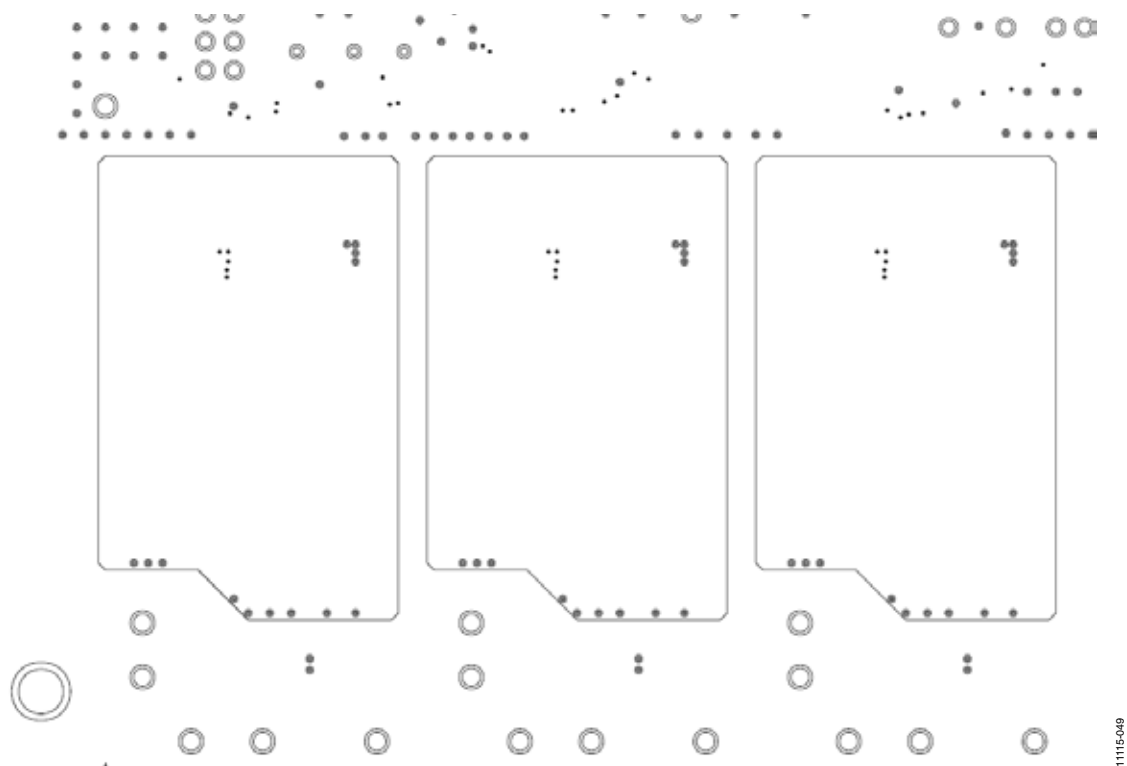
图61. 4层电路板：第3层
