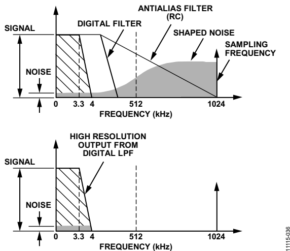
图26. 模拟调制器中通过过采样和噪声整形实现降噪
