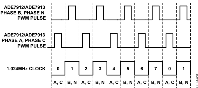
图49. 使用四个ADE7912/ADE7913器件的三相电表的EMI管理
