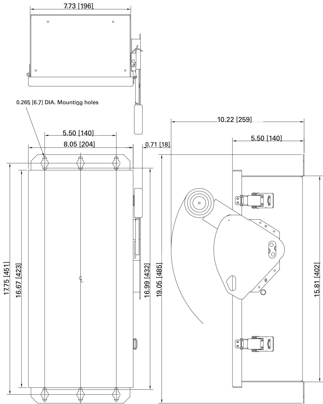
Dimensions FO
