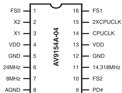
16-SOIC 9154A-04CS16
