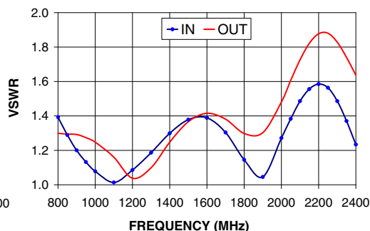
ZX60-2411BM+ VSWR
