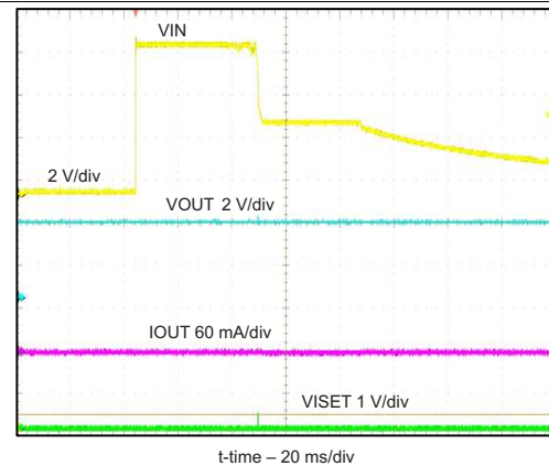
图 4. OVP 7-V Adaptor
