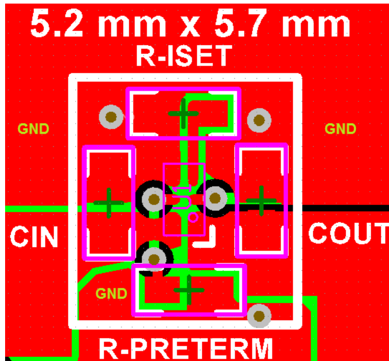
图 28. Board Layout
