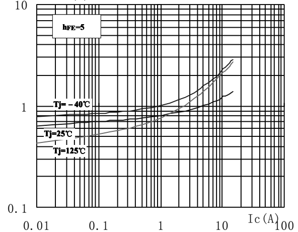
V_{bes} - I_c
