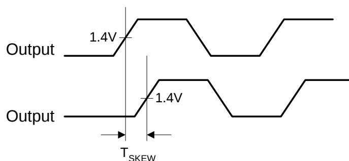
Output - Output Skew
