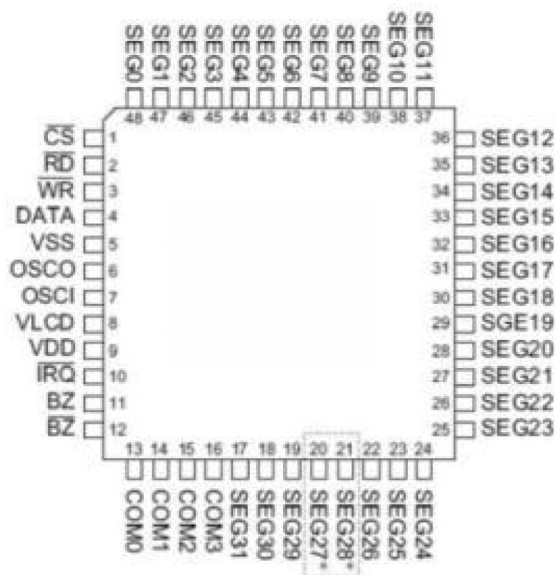
1621B 48LQFP-A
