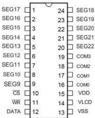
1621B 24SOP-A/SSOP-A
