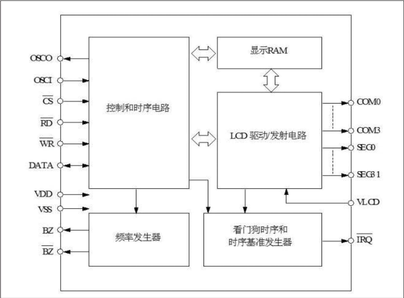
功能框图
