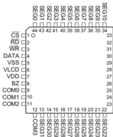
1621B 44LQFP-A
