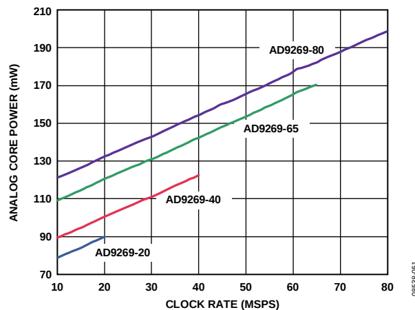
图56. 模拟内核功耗与时钟速率的关系
