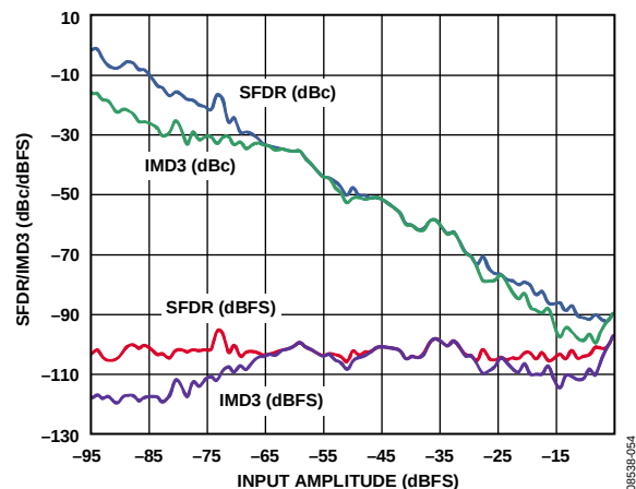
图11. 双音SFDR/IMD3与输入幅度( A_{IN} )的关系 ( f_{IN1} = 28.3\text{ MHz} 、 f_{IN2} = 30.6\text{ MHz} )
