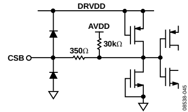
图 36. 等效CSB输入电路
