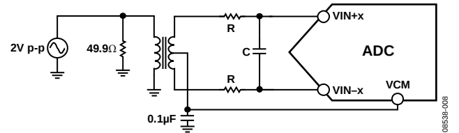
图41. 差分变压器耦合配置
