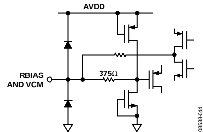
图35. 等效RBIAS、VCM电路
