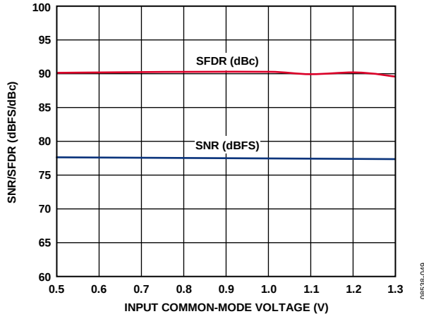
图39. SNR/SFDR与输入共模电压的关系 ( f_{IN} = 32.5 \text{ MHz} , f_s = 80 \text{ MSPS} )
