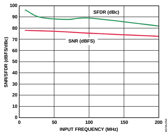
图22. AD9269-65 SNR/SFDR与输入频率( A_{IN} )的关系 (2 V峰峰值满量程)
