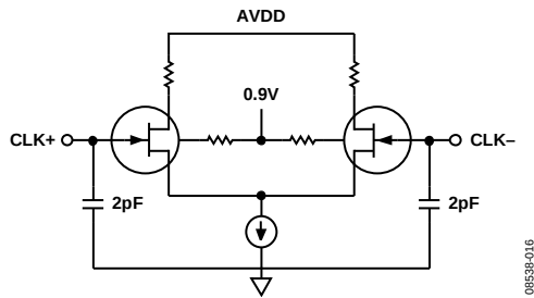
图48. 等效时钟输入电路
