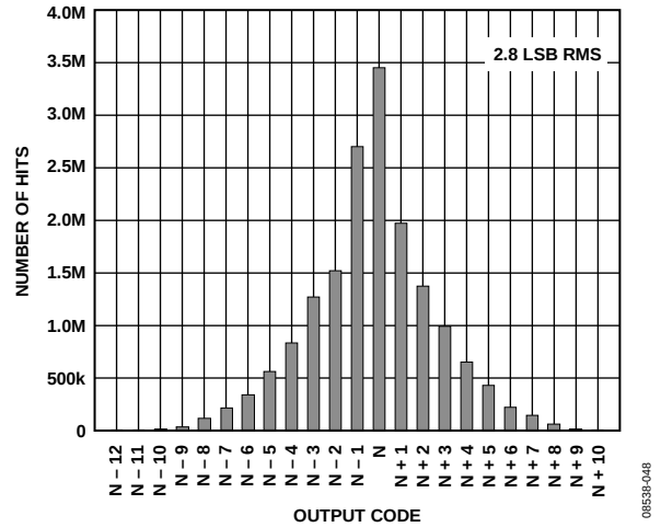
图16. 接地输入直方图
