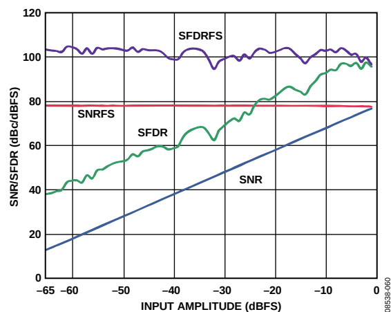
图21. AD9269-65 SNR/SFDR与输入幅度( A_{IN} )的关系( f_{IN} = 9.7\text{ MHz} )
