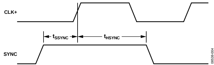
图4. SYNC输入时序要求
