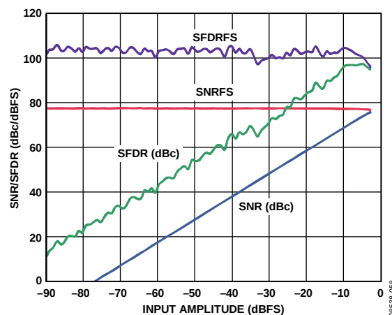
图28. AD9269-20 SNR/SFDR与输入幅度( A_{IN} )的关系 ( f_{IN} = 9.7\text{ MHz} )
