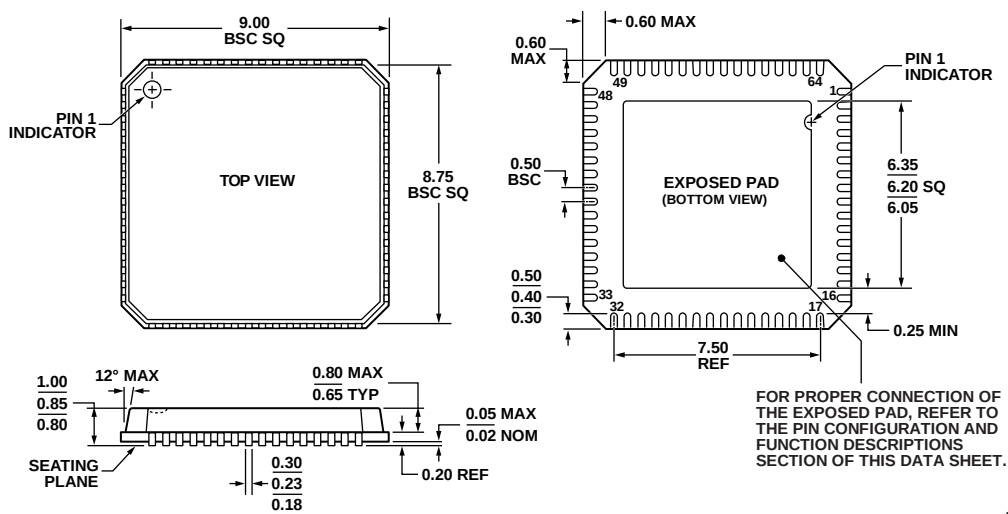
图60. 64引脚|脚架构芯片级封装[LFCSP_VQ], 9 mm x 9 mm超薄四方体(CP-64-4), 尺寸单位: mm
