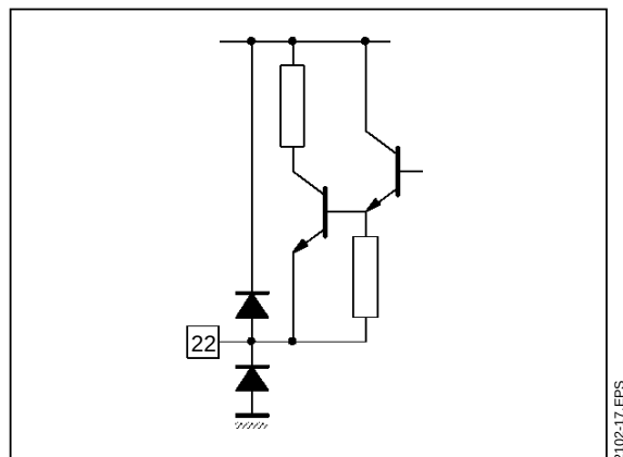
Figure 15 : Pin 22 (DLO)
