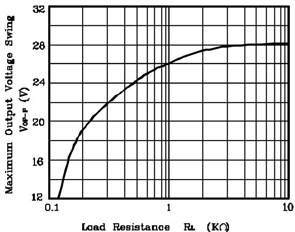
Fig. 5 V_{OP-P} - R_L
