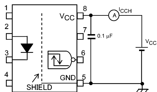
Fig. 12.1.4 I_{CCH} Test Circuit
