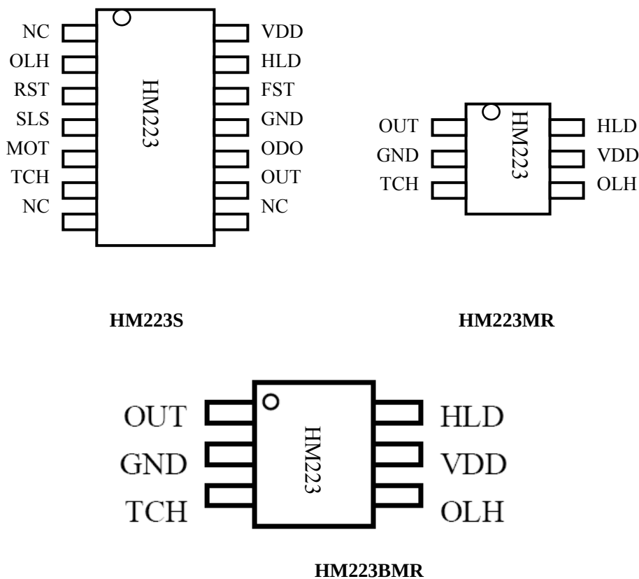
图 1 封装示意图
