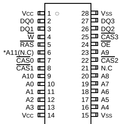
• KM44C40(1)05CS
