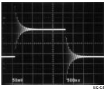
Small-Signal Transient, AV = 1, CL = 1000pF
