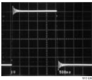
Large-Signal Transient, AV = 1, CL = 1000pF
