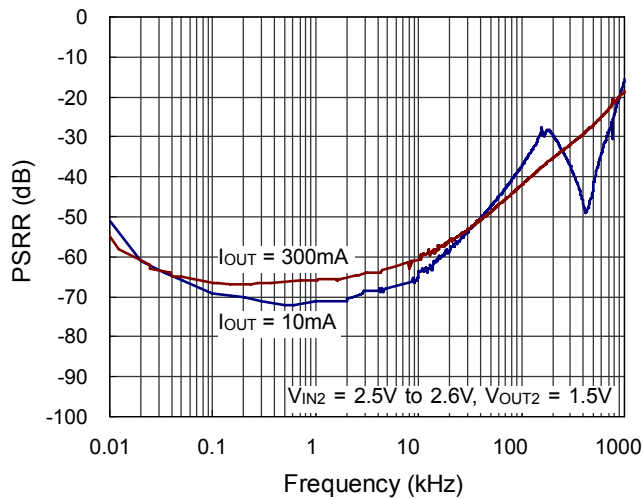
LDO1 PSRR
