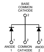
D 2 PAK
