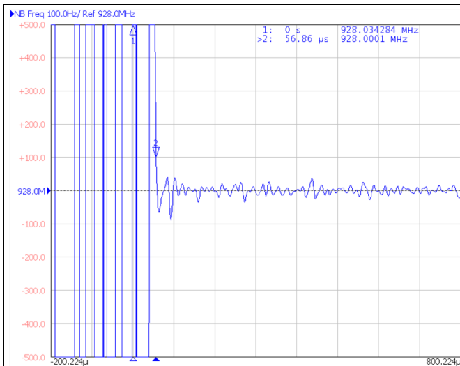
Figure 67. F1 to F2 Switching Time
