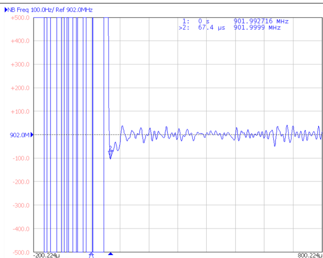
Figure 68. F2 to F1 Switching Time
