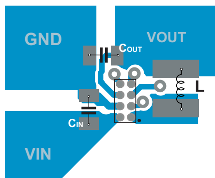
图 28. Recommended PCB Layout
