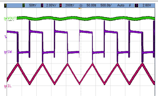
图 21. PWM Mode Operation
