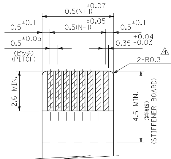
適用FPC推奨寸法 APPLICABLE FPC RECOMMENDED DIMENSION （仕上がり厚さ：0.3±0.03） （THICKNESS:0.3±0.03）
