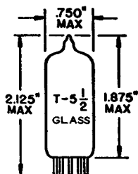
BASE 7 PIN MINIATURE BUTT JEDEC E7-1
