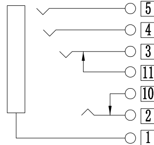
电路图
