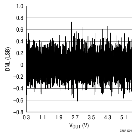
VOUT_COMMAND DNL
